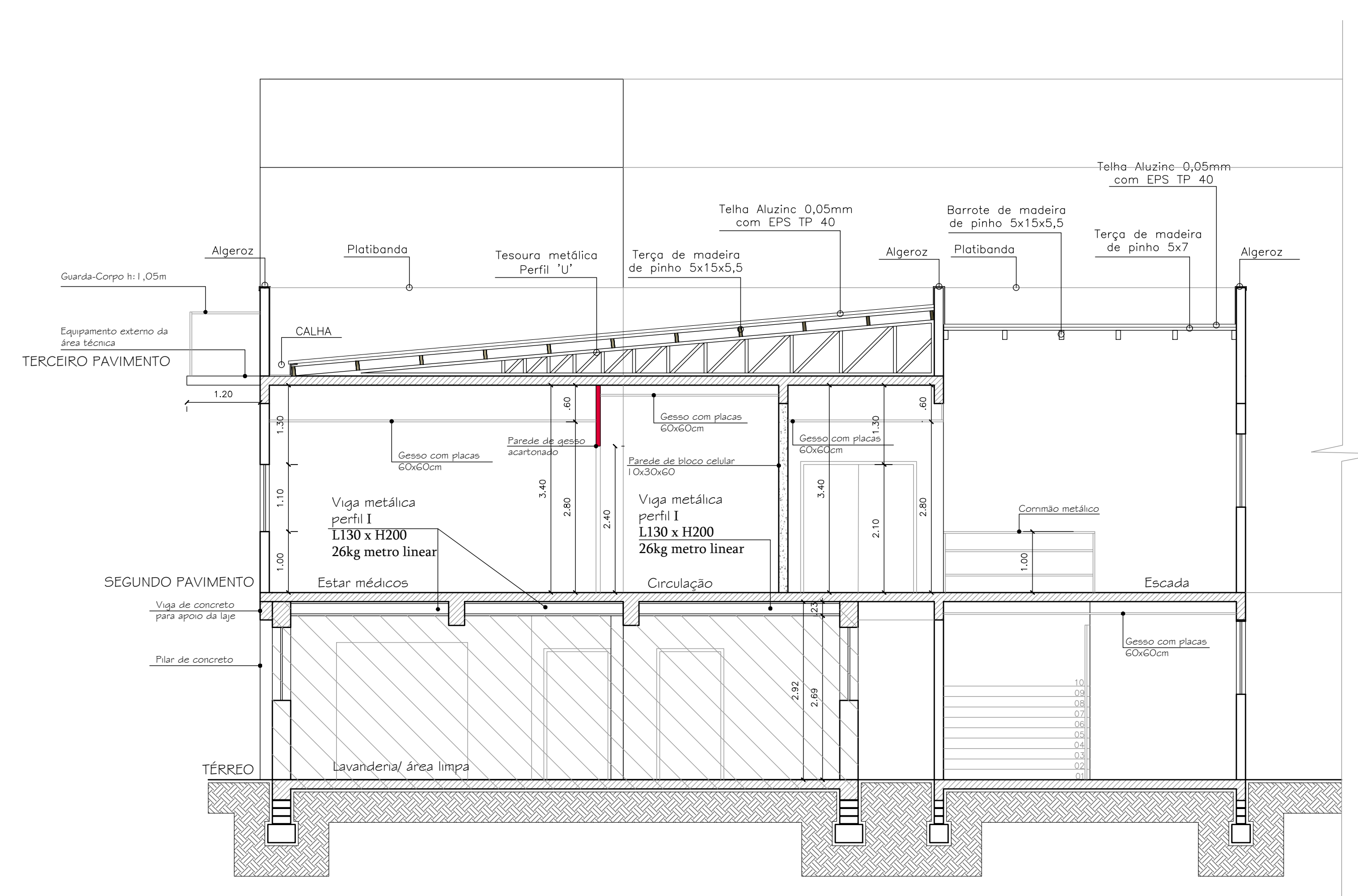
2 CORTE BB
